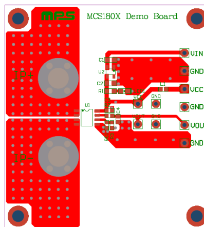
Top Layer
