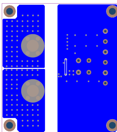
Bottom Layer
