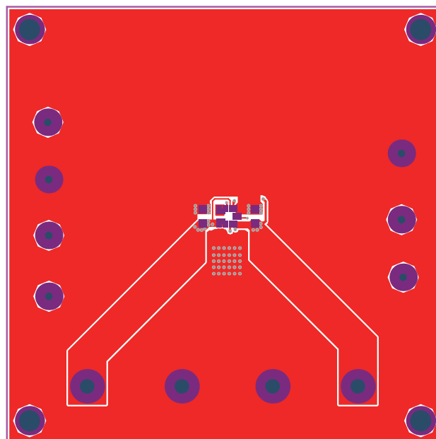
Figure 4—Top Layer
