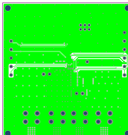
Figure 4— Inner Layer 2
