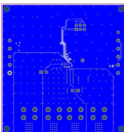
Figure 5—Bottom Layer
