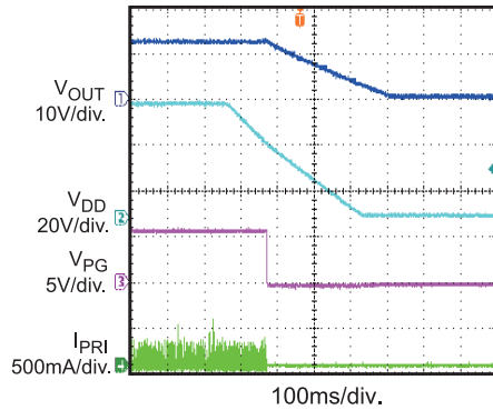
V DD Shutdown
