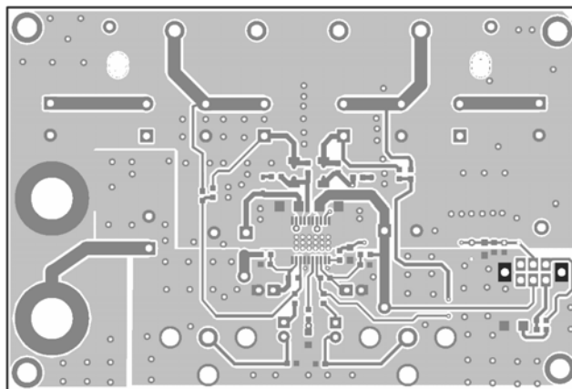
Figure 2—Top Layer
