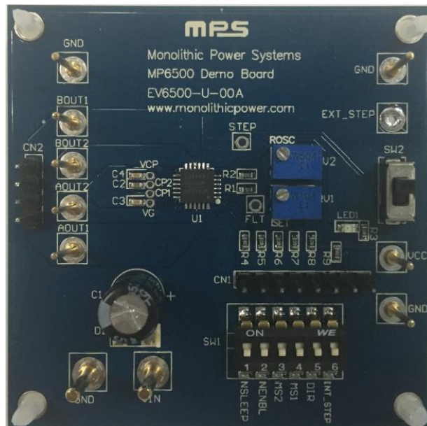
(LxWxH) 6.35cmx6.35cmx1cm
