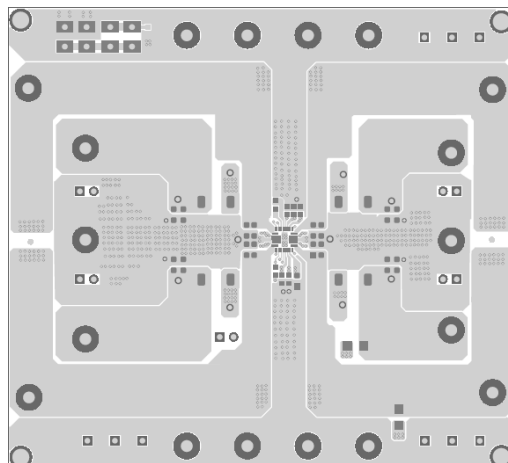
Figure 2—Top Layer
