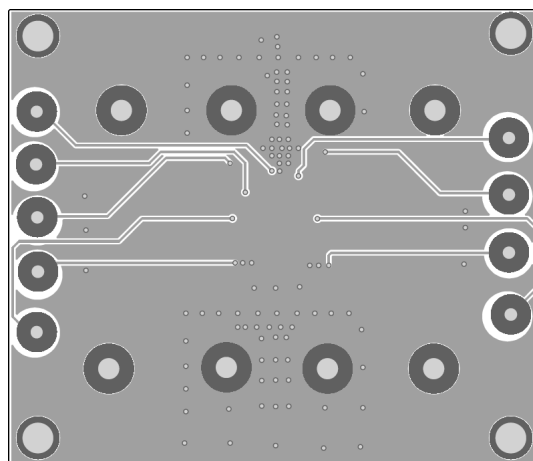
Figure 5—Bottom Layer
