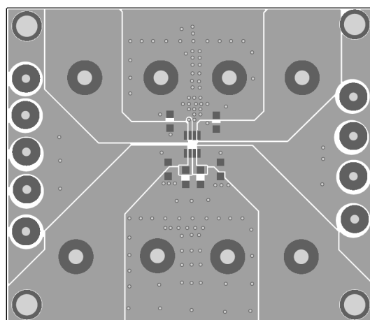
Figure 2—Top Layer
