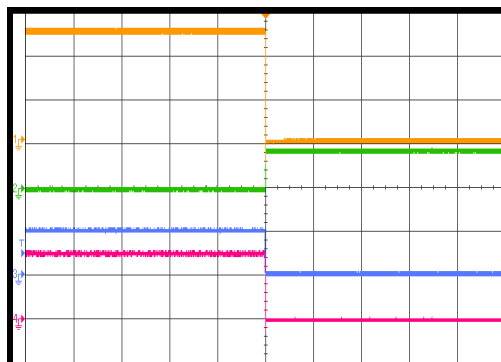
EN shutdown
