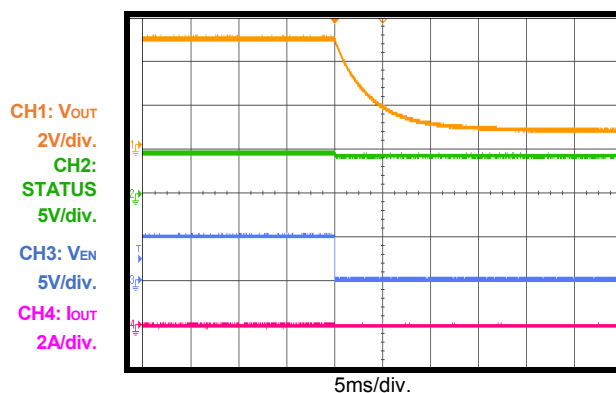
EN shutdown
