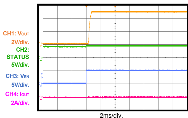
EN start-up
