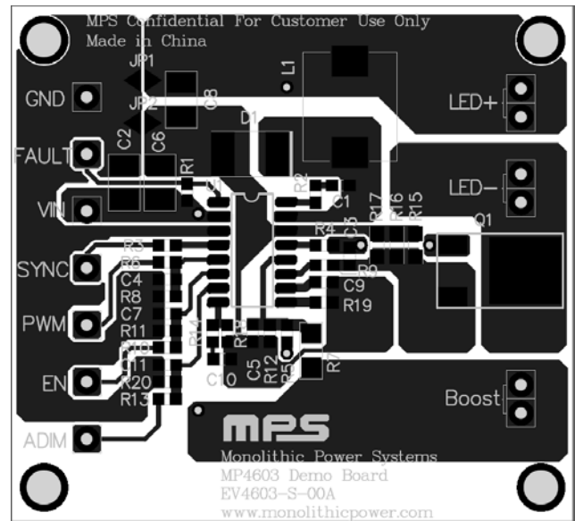
Figure 2—Top Layer
