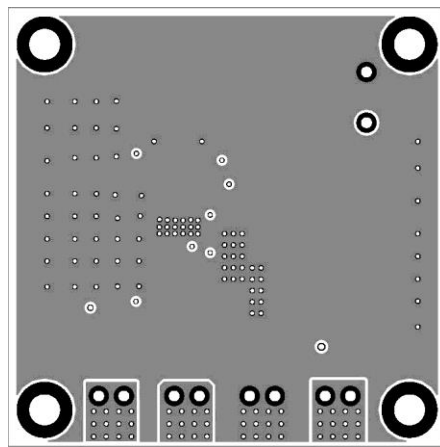
Figure 5—Bottom Layer
