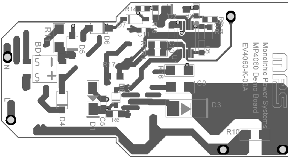
Figure 3—Bottom Layer
