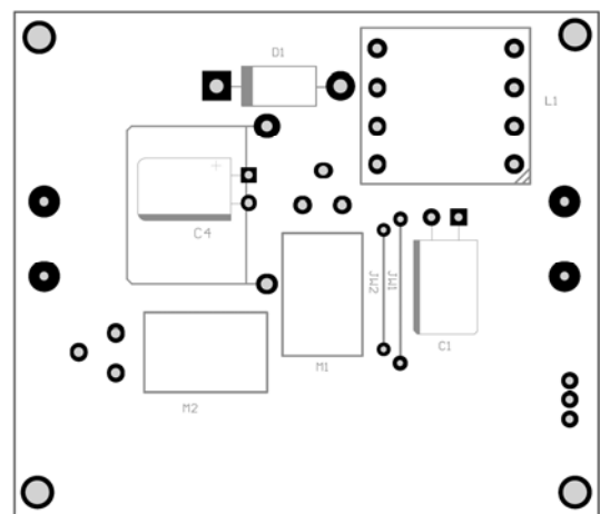
Figure 4—Bottom Layer
