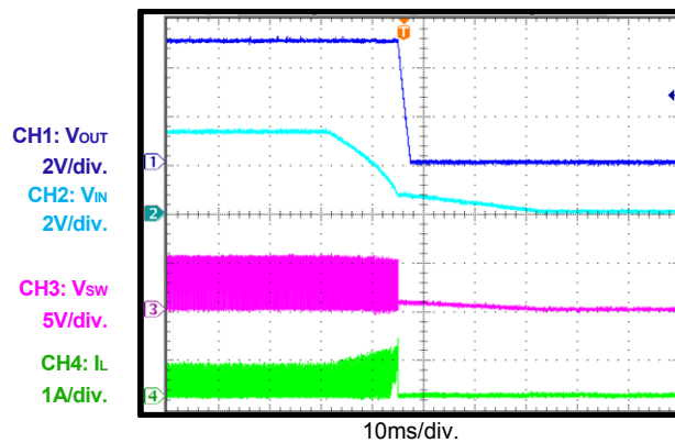
VIN Shutdown
