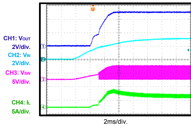
VIN Start-Up
