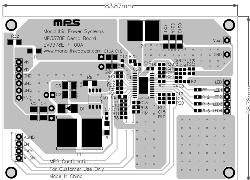
Figure 1—Top Layer
