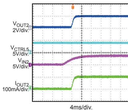
VIN On I_{OUT2} = 0.1A
