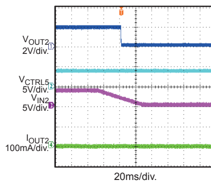
VIN Off I_{OUT2} = 0A
