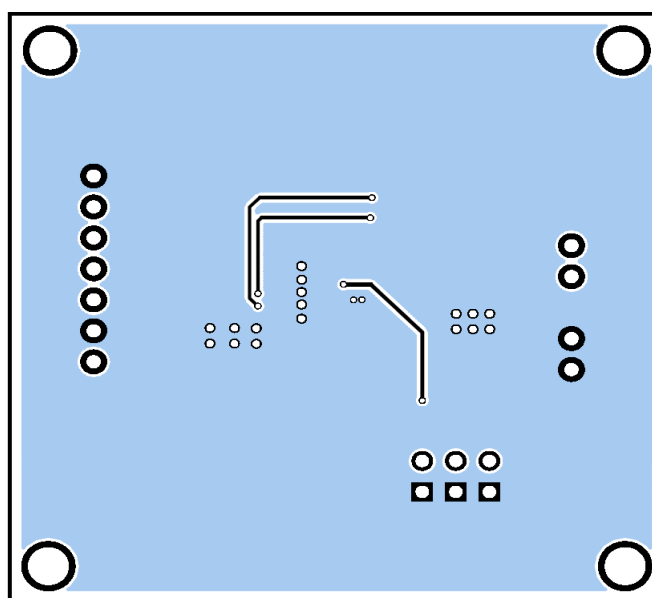
Figure 3—Bottom Layer
