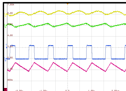
Input/Output ripple
