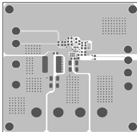
Figure 2—Top Layer
