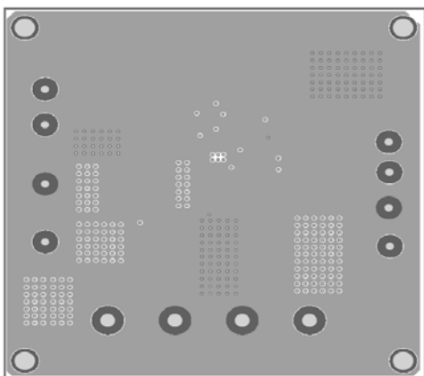
Figure 1—Top Silk Layer
