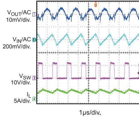
Input/Output Ripple
