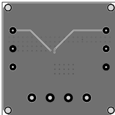
Figure 4—Bottom Layer
