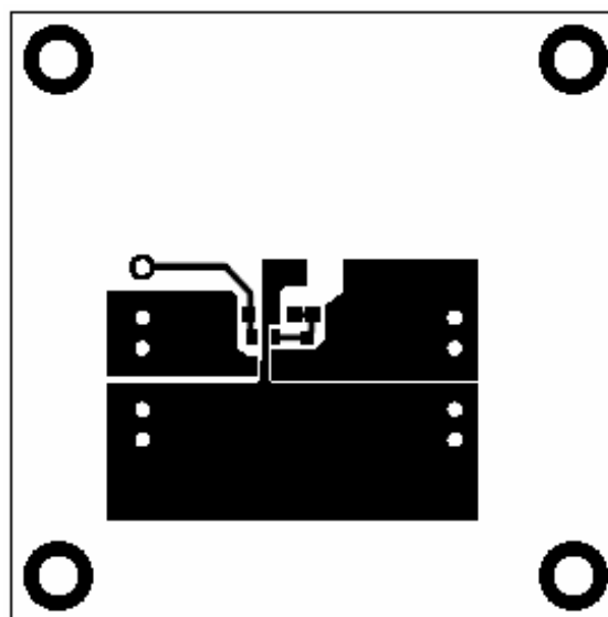
Figure 2—Top Layer
