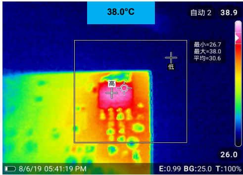
Thermal V_{IN}=85V_{AC}
