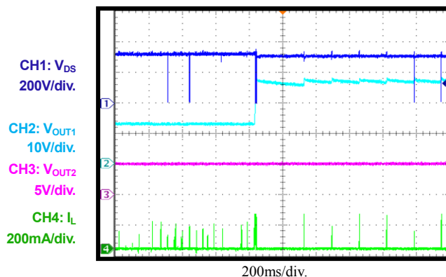
V_{OUT1} OVP
