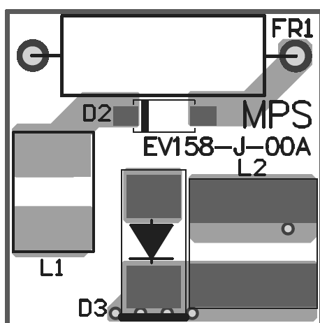
Figure 3—Bottom Layer
