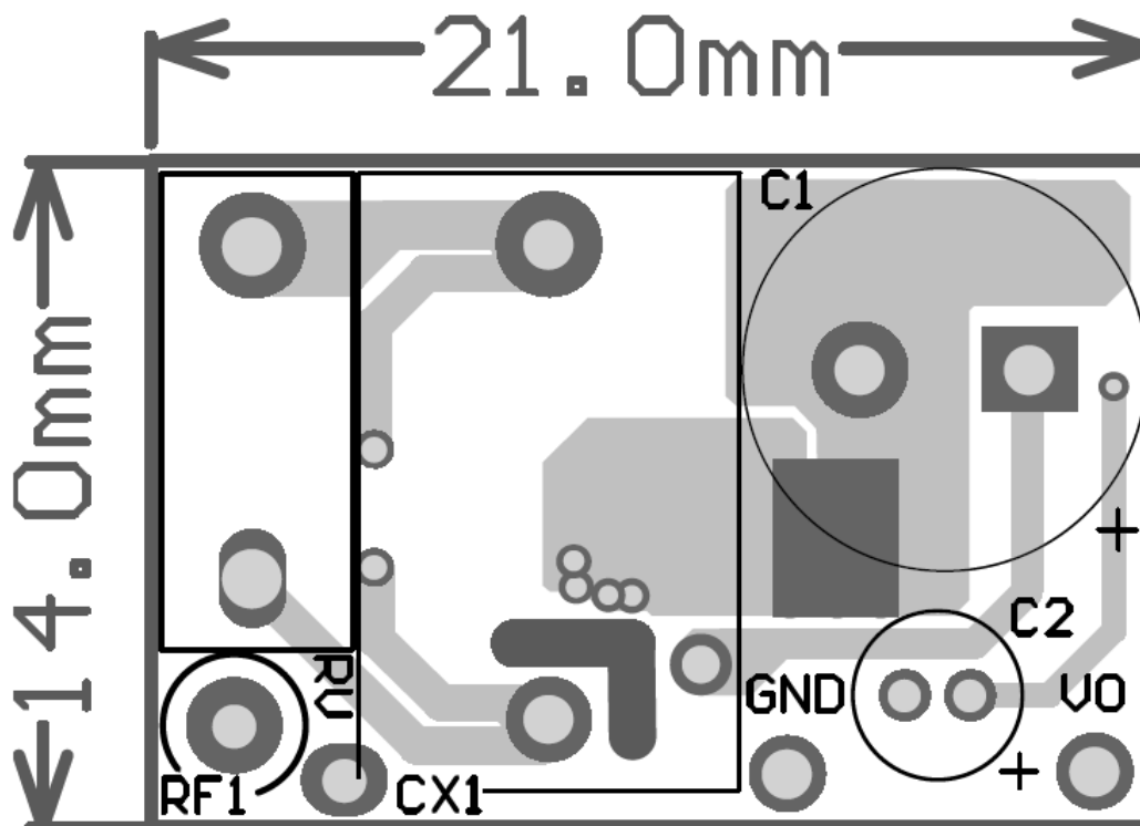
Figure 2 — Top Layer
