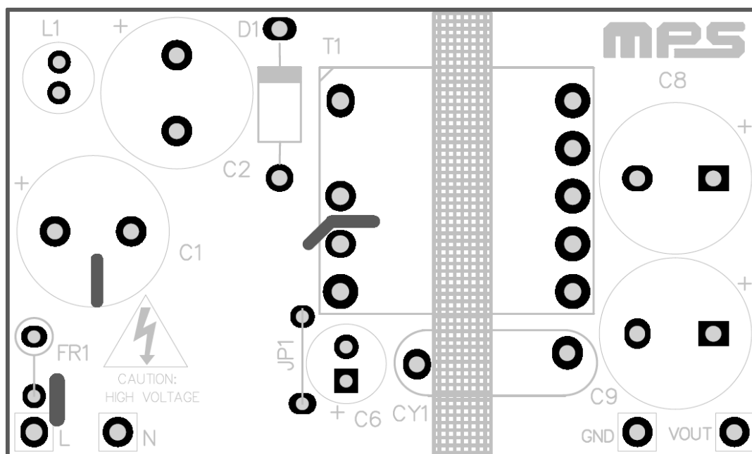
Figure 2—Top Layer
