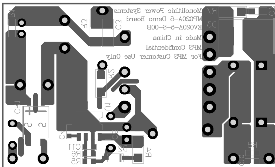
Figure 3—Bottom Layer
