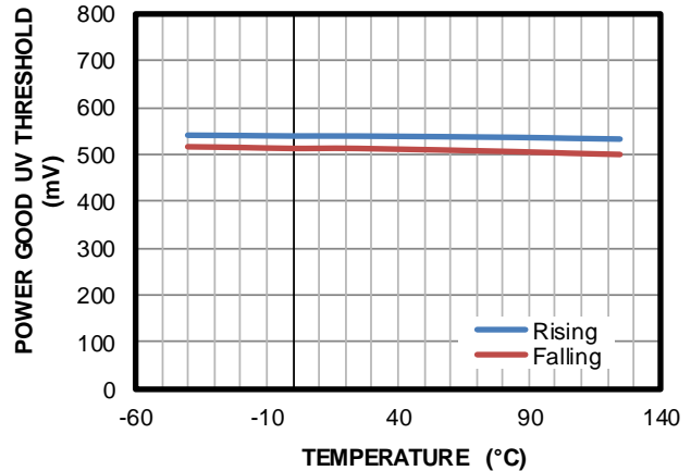
电源正常输出指示欠压阈值 vs. 温度
