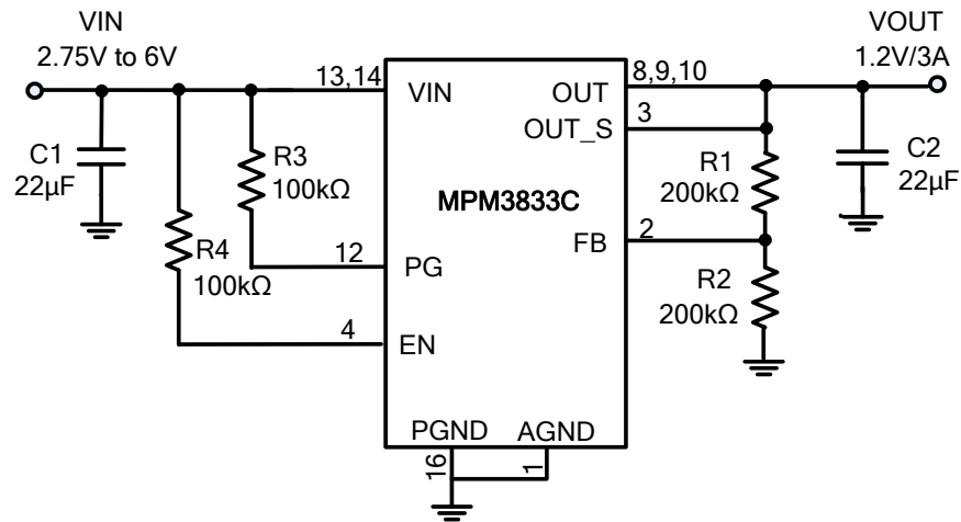
图 4: MPM3833C 典型应用电路
