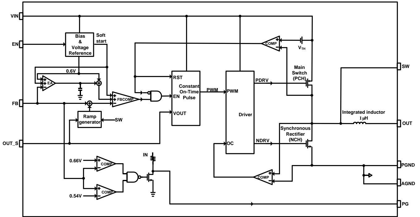
图 1: 功能框图
