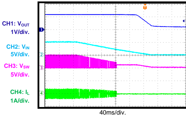
V_{IN} 关断 I_{OUT} = 0A
