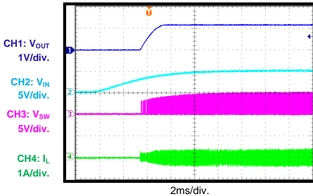
V_{IN} 上电 I_{OUT} = 0A
