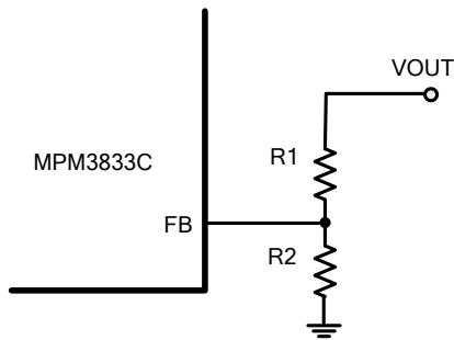
图 2: 反馈网络
