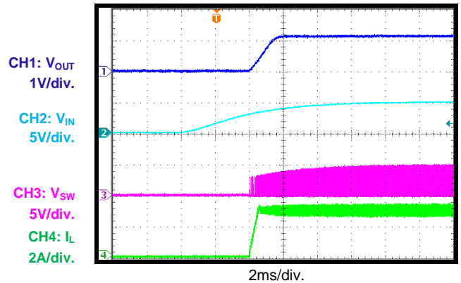
V_{IN} 上电 I_{OUT} = 3A
