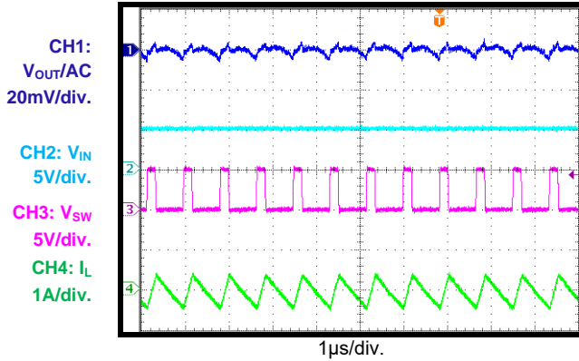
稳态 I_{OUT} = 0A
