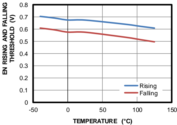
EN 上升和下降阈值 vs. 温度
