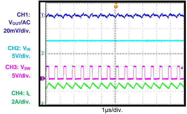
稳态 I_{OUT} = 3A
