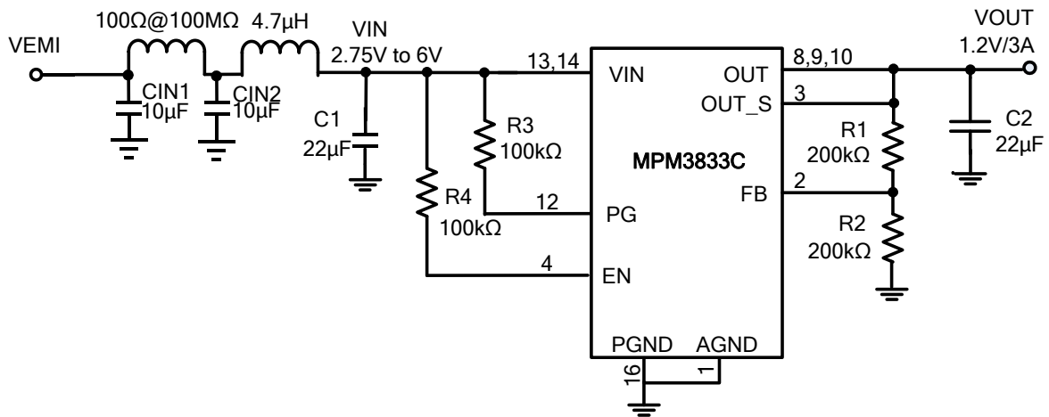
图 6: MPM3833C EMI 测试电路
