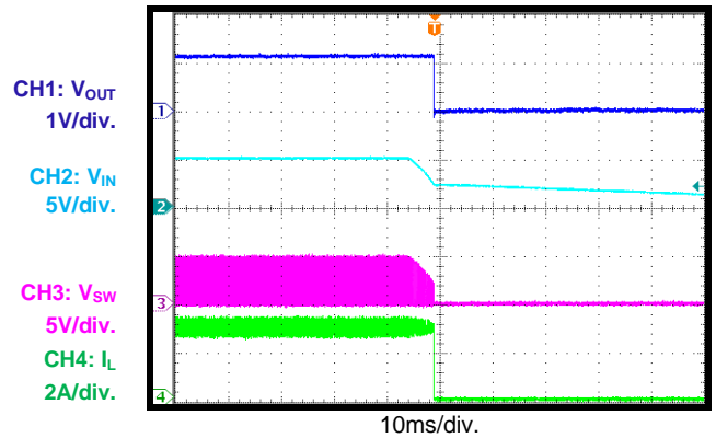
V_{IN} 关断 I_{OUT} = 3A
