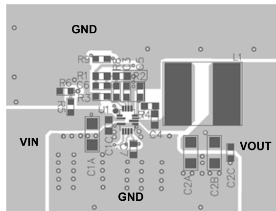
Top Layer
