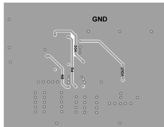
Bottom Layer
