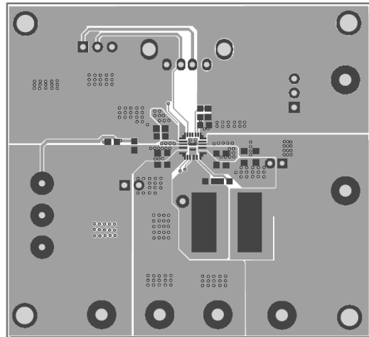
Figure 2—Top Layer
