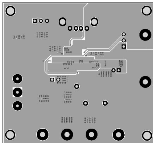
Figure 5—Bottom Layer
