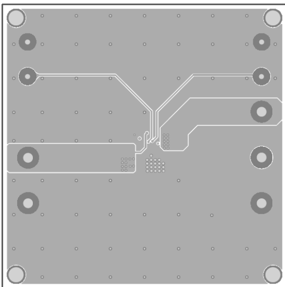
Figure 3-IN2 Layer
