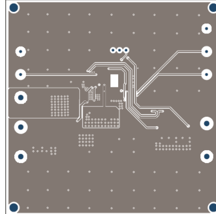
Figure 4— Middle Layer 2
