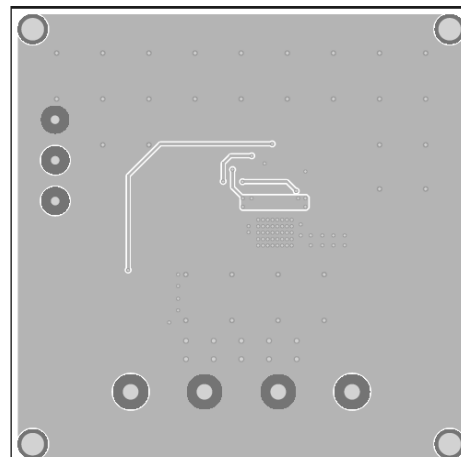
Figure 5—Bottom Layer
