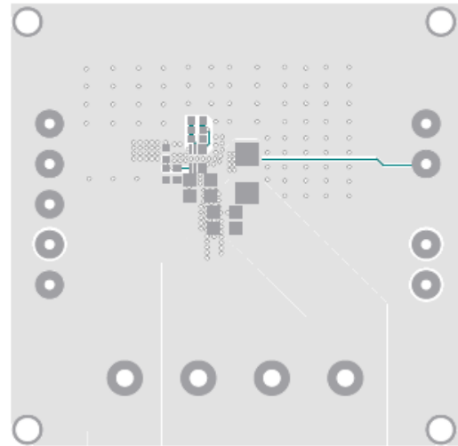
Figure 2—Top Layer
