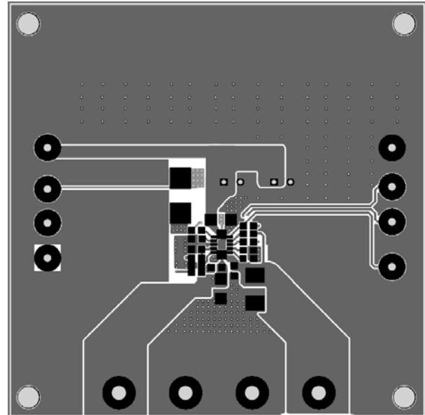
Figure 2—Top Layer
