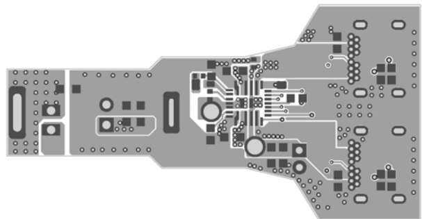
Figure 6—Bottom Layer
