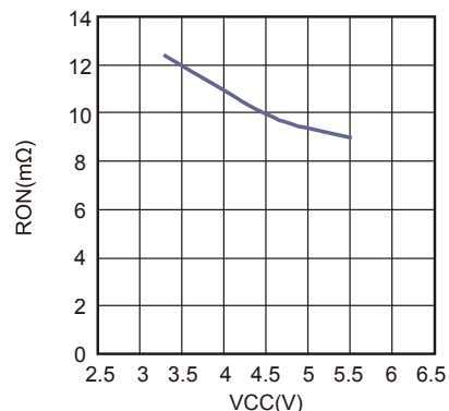
Rds_on vs.Vcc
