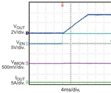
Enable Startup
