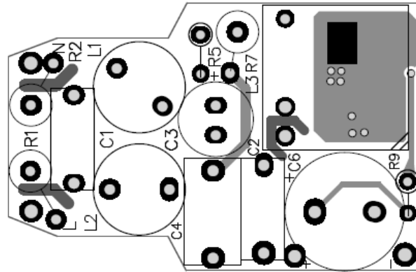
Figure 2—Top Layer
