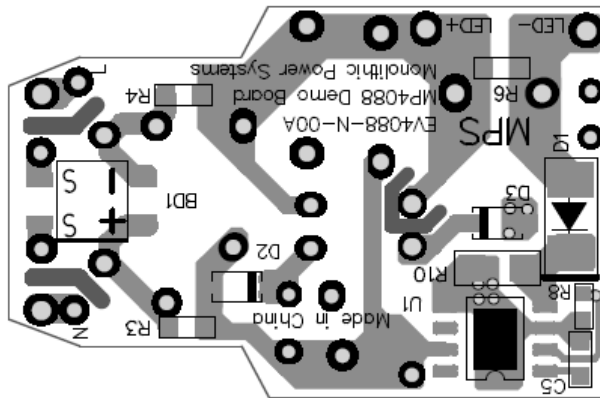
Figure 3—Bottom Layer
