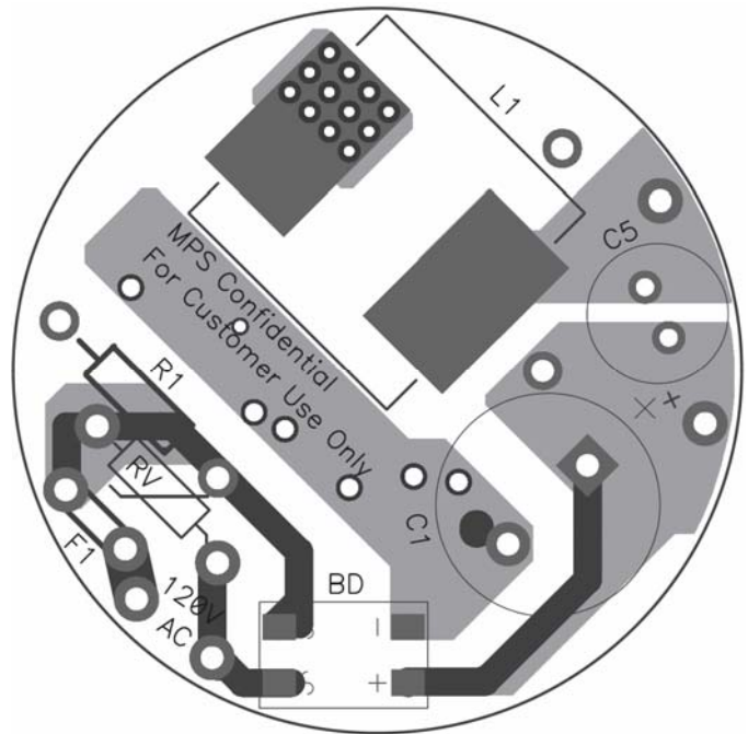
Figure 4—Bottom Layer
