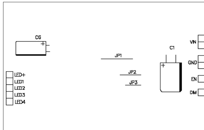
Figure 2—Bottom Layer
