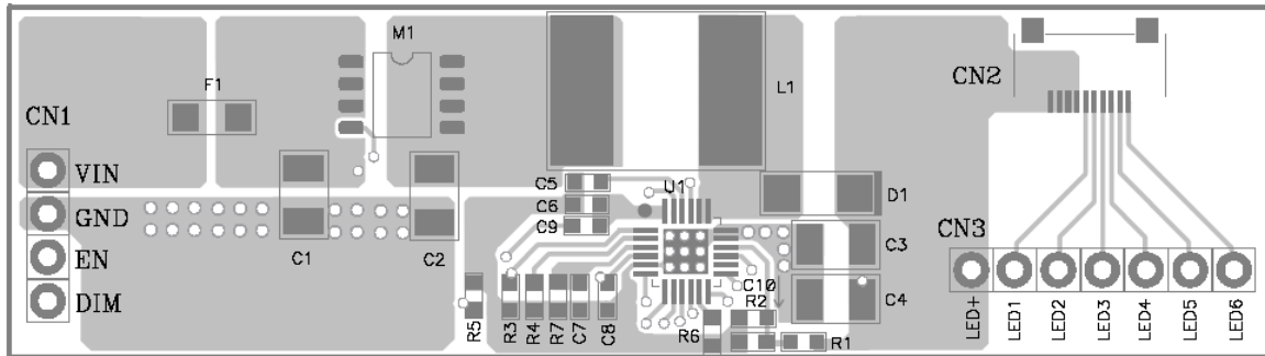
Figure 1—Top Layer
