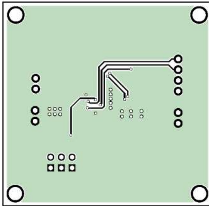
Figure 3—Bottom Layer
