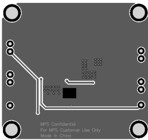
Figure 3—Bottom Layer
