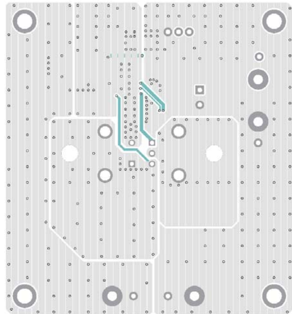
Figure 4—Bottom Layer
