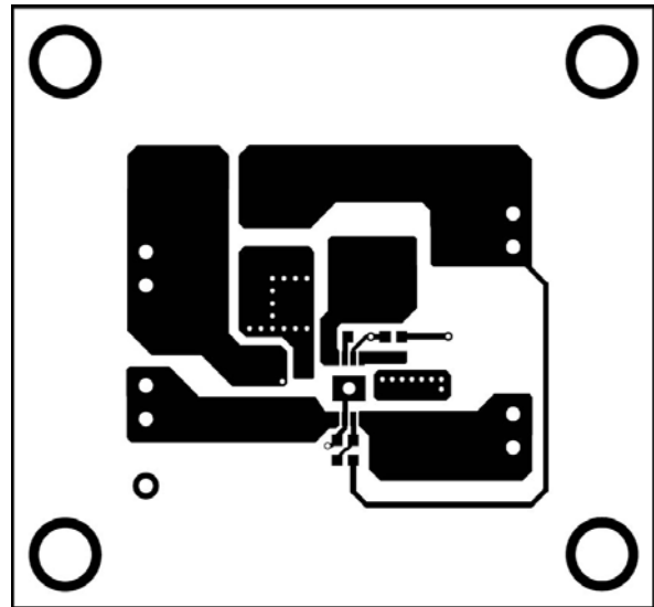
Figure 2—Top Layer
