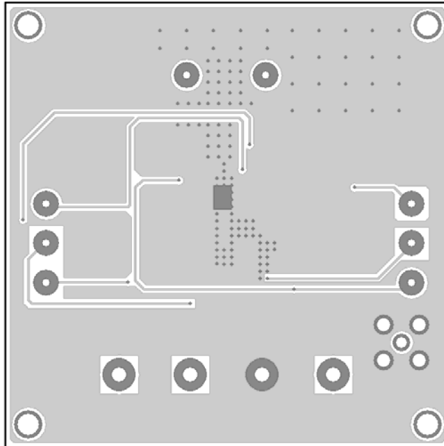
Figure 3—Bottom Layer
