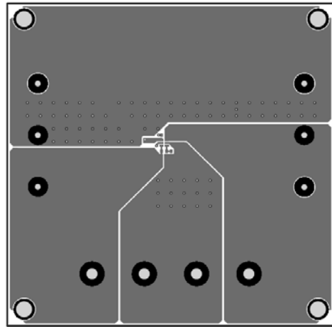
Figure 3—Top Layer
