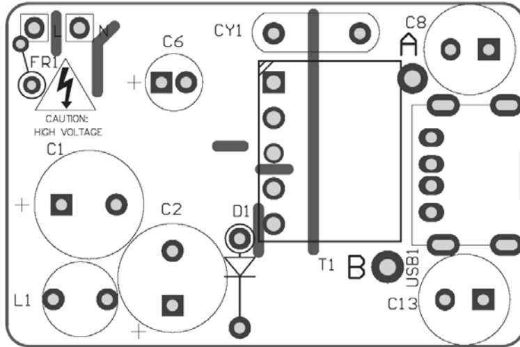
Figure 2—Top Layer
