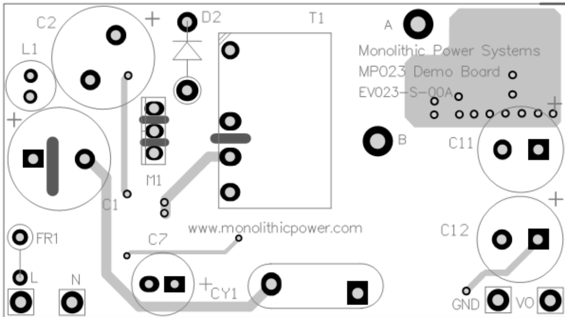
Figure 2—Top Layer
